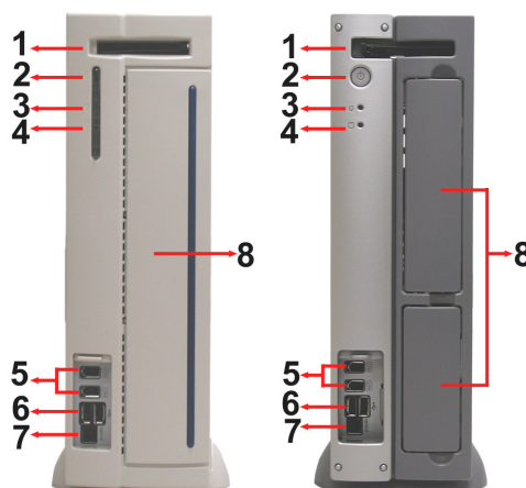
slika 1.1 Prednja strana kućíšta (izgled ovisi o modelu računala).
